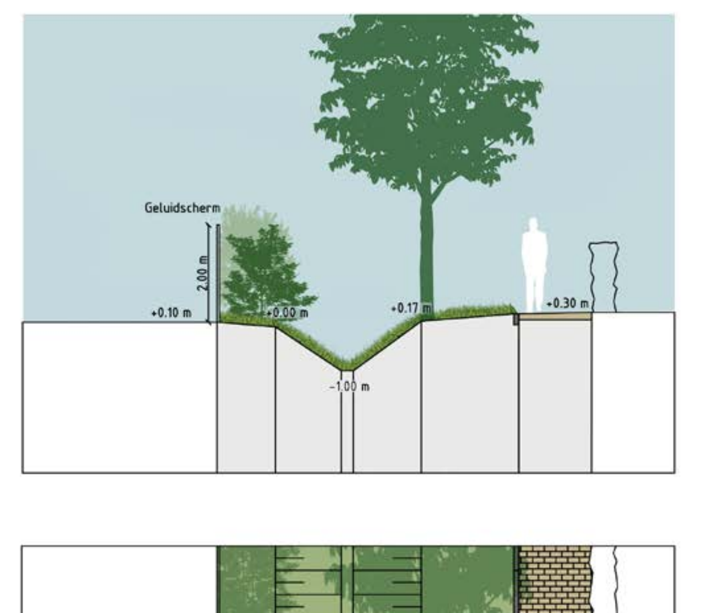
E: profiel van greppel achter transport-bedrijf Boer
