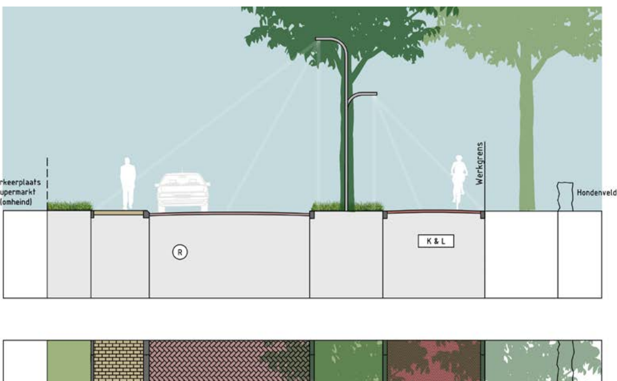
C: profiel van de entreestraat vanaf de Grafhorsterweg
