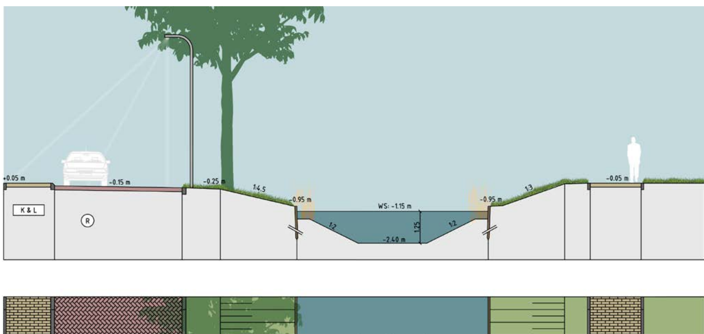
A: profiel van de hoofdstraat met laan en watergang
