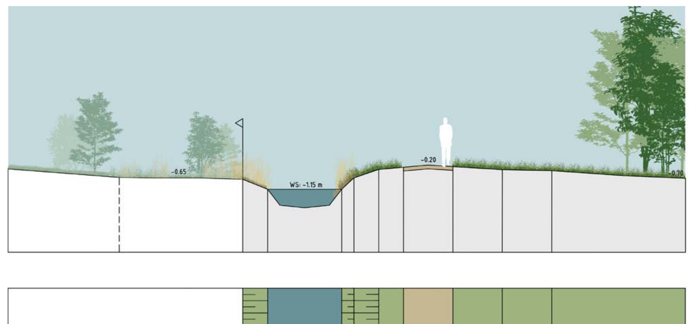
B: profiel van de Ringdijk met wandelroute aan de noordoost kant
